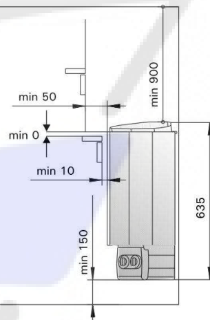
Obr. 6 Bezpečnostní vzdálenosti od kamen
